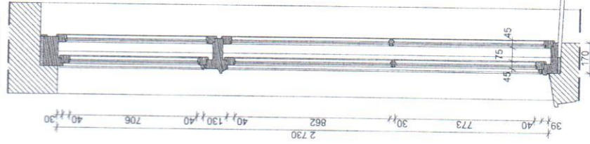
Przekrój B-B
