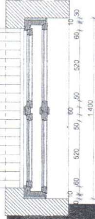
Przekrój A-A
